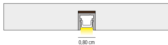
INSTALLAZIONE AD INCASSO RECESSED INSTALLATION
