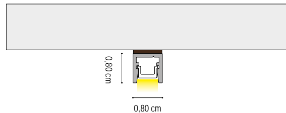
INSTALLAZIONE SU SUPERFICI ORIZZONTALI INSTALLATION ON HORIZONTAL SURFACES
