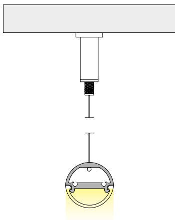
INSTALLAZIONE A SOSPENSIONE SUSPENSION
