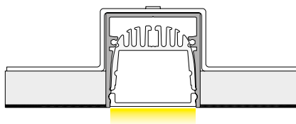
INSTALLAZIONE A INCASSO IN CARTONGESSO RECESSED INSTALLATION IN PLASTERBOARD
