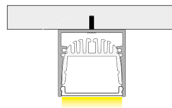
INSTALLAZIONE A SOFFITTO CEILING INSTALLATION
