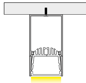
INSTALLAZIONE A SOFFITTO CEILING INSTALLATION
