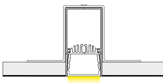
INSTALLAZIONE A INCASSO IN CARTONGESSO RECESSED INSTALLATION IN PLASTERBOARD
