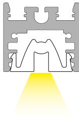
VERSIONE SPOT (15°) SPOT VERSION (15°)
