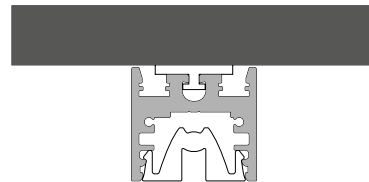
INSTALLAZIONE CON STAFFE MAGNETICHE SU SUPERFICIE METALLICA ORIZZONTALE INSTALLATION WITH MAGNET ON HORIZONTAL METAL SURFACE
