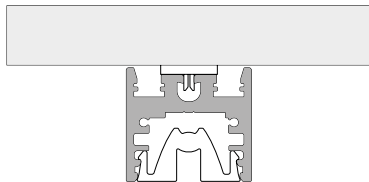
INSTALLAZIONE CON CLIP IN POLICARBONATO SU SUPERFICIE ORIZZONTALE INSTALLATION WITH POLYCARBONATE CLIP ON HORIZONTAL SURFACE
