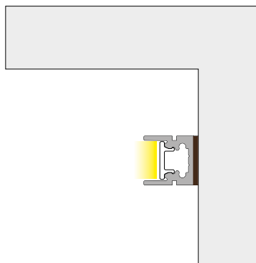
INSTALLAZIONE SU SUPERFICI VERTICALI INSTALLATION ON VERTICAL SURFACES
