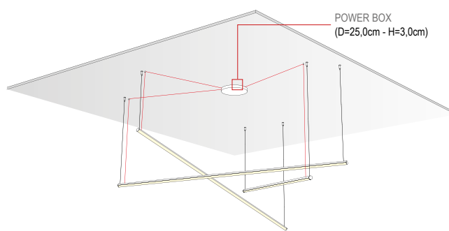
COSTELLAZIONE CON BOX COSTELLAZIONE WITH POWER SUPPLY BOX
