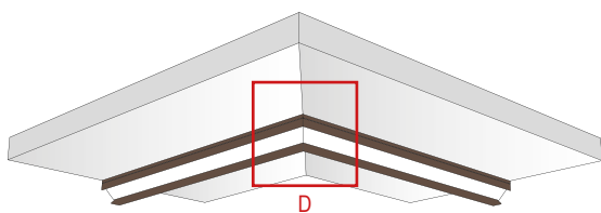
D) TAGLIO ANGOLARE - SUPERFICIE ORIZZONTALE - TIPO D D) CORNER CUT - HORIZONTAL SURFACE - TYPE D
